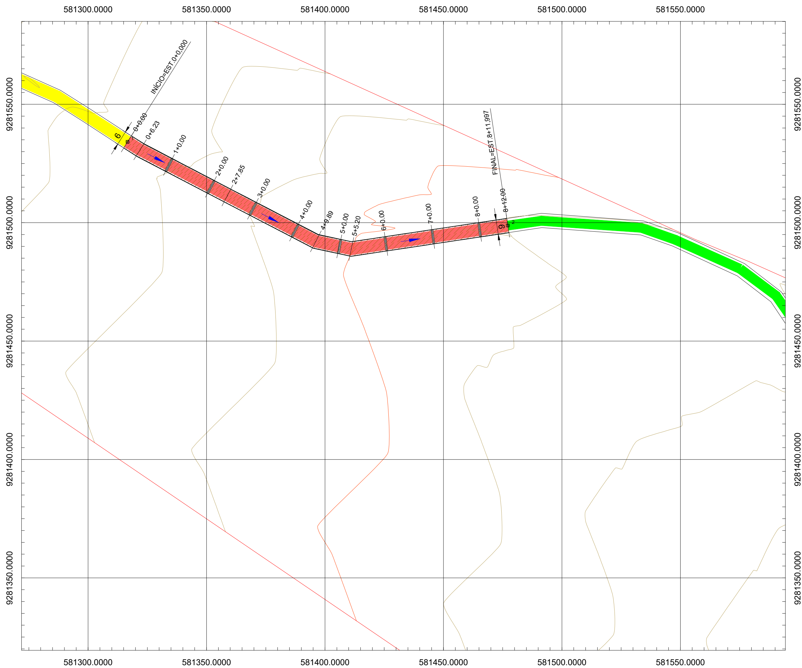
Planimetria Escala 1:1000
