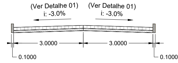
Seção Transversal Tipo Escala 1:100
