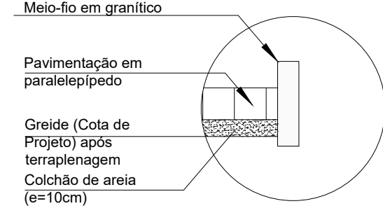
Detalhe 01 Escala 1:25
